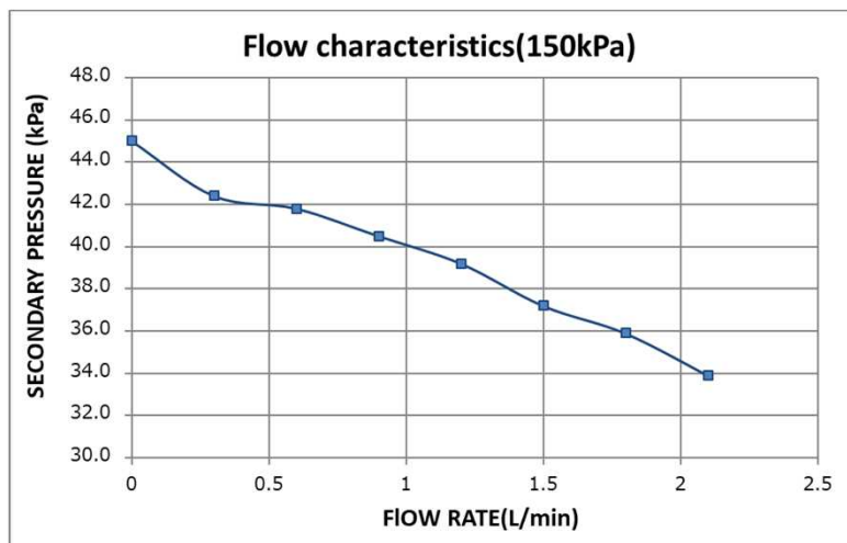
【流量特性】
