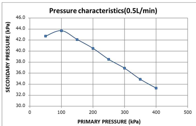
【圧力特性】
